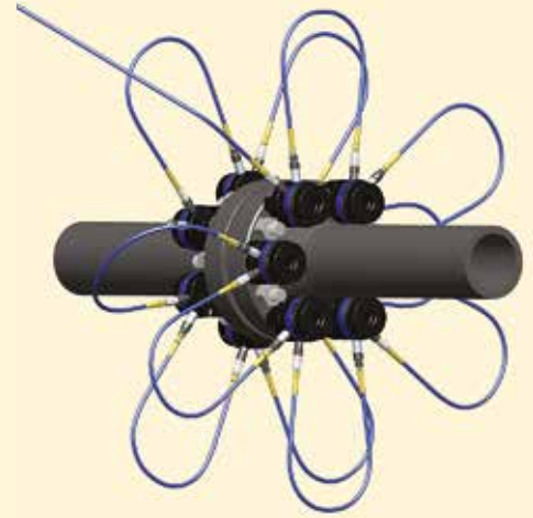
Configuration au moyen d'une procédure de mise en tension 100% Tous les goujons sont tendus simultanément.
