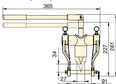
Rétraction et déploiement de l'outil à l'aide d'une petite barre d'écartement (Ø 16 mm)
