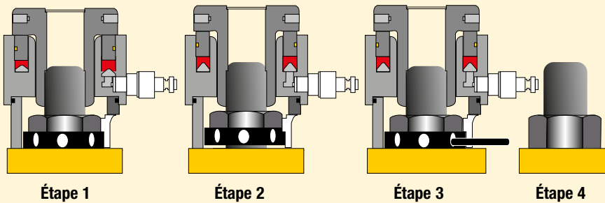
Configuration au moyen d'une procédure de mise en tension 100% Tous les goujons sont tendus simultanément.
